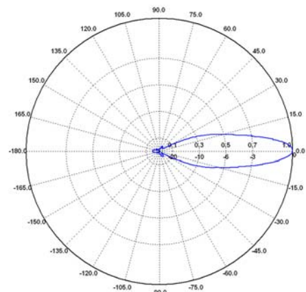
H-plane / H-Plane 8 GHz
