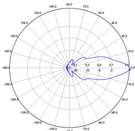
E-plane / E-Plane 8 GHz
