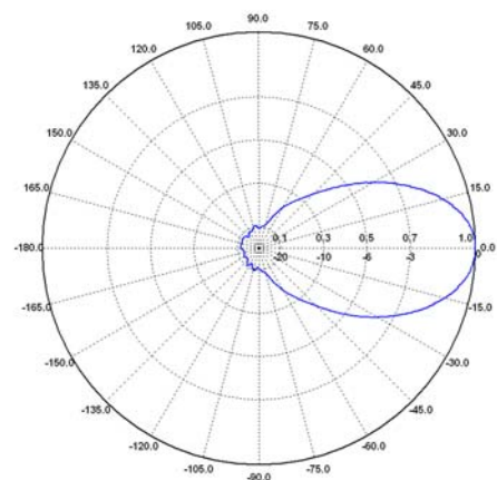
H-plane / H-plane 2 GHz
