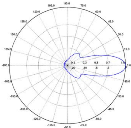
E-plane / E-Plane 4 GHz
