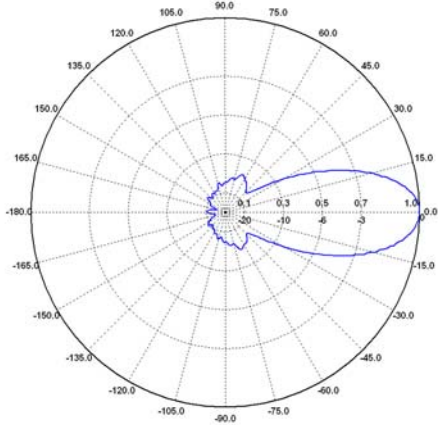
E-plane / E-Plane 3 GHz
