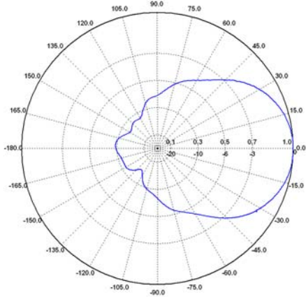
E-plane / E-Plane 1 GHz
