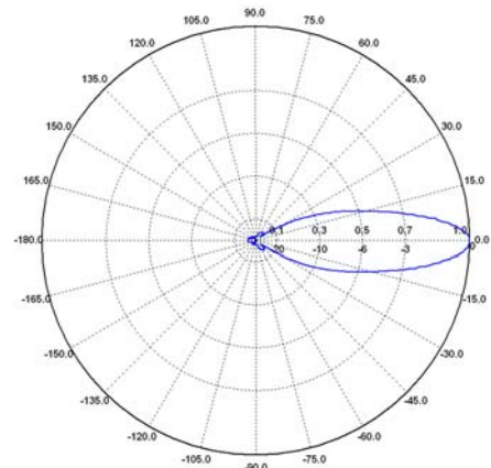
H-plane / H-Plane 7 GHz
