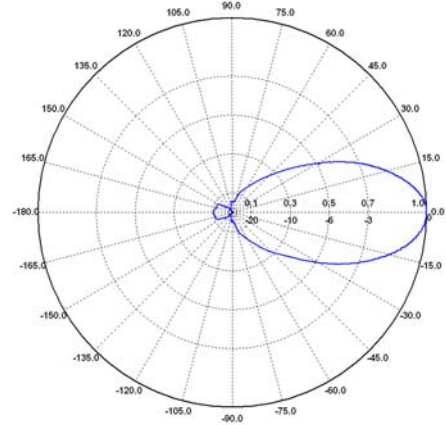
H-plane / H-plane 3 GHz
