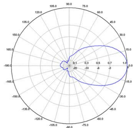
H-plane / H-Plane 1.5 GHz
