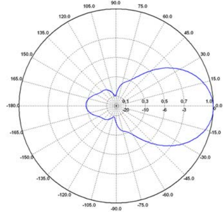
H-plane / H-plane 1 GHz
