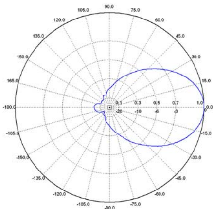
E-plane / E-Plane 1.5 GHz
