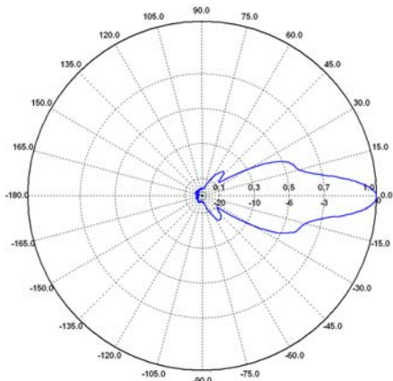
E-plane / E-Plane 7 GHz
