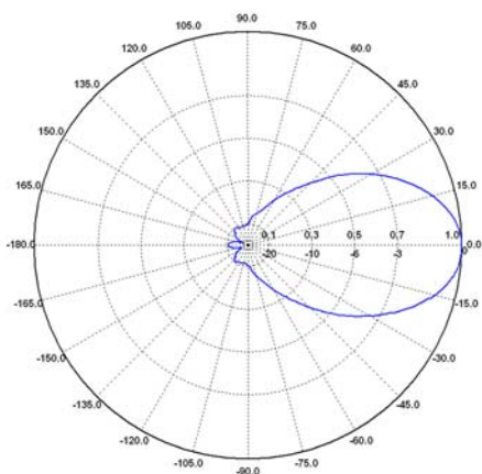
E-plane / E-Plane 2 GHz
