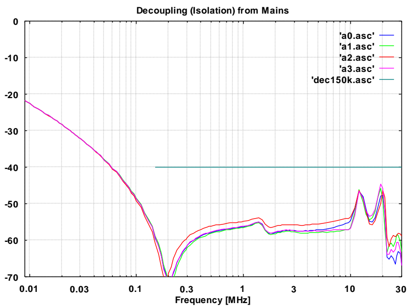
Abb. 7: Entkopplung vom Speisernetz, BNC mit 50 Ω Abschluss Fig. 7: Decoupling from supply net, BNC terminated with 50 Ω
