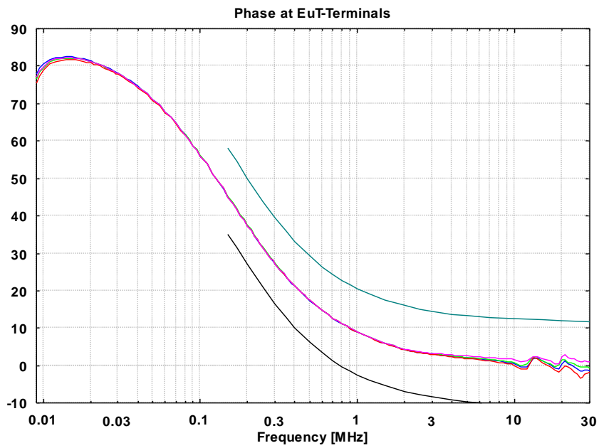
Abb. 6 Phase an den Prüflingsklemmen, BNC mit 50 Ω Abschluss Fig. 6: Phase at the connector for DuT, BNC terminated with 50 Ω
