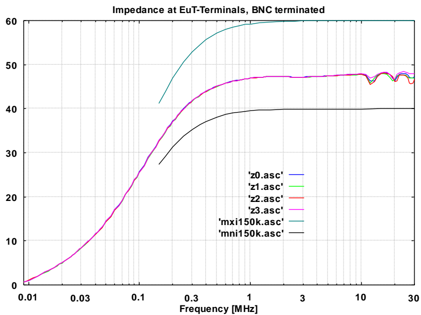
Abb. 5: Impedanz an den Prüflingsklemmen), BNC mit 50 Ω Abschluss Fig. 5: Impedance of connector for DuT, BNC terminated with 50 Ω
