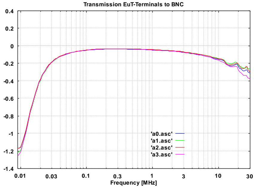
Abb. 4: Transmission Prüflingsklemmen - BNC Fig. 4: Transmission - BNC
