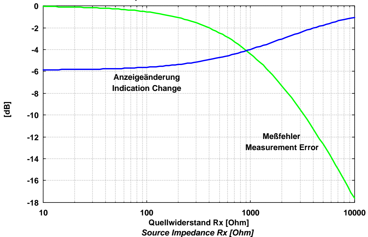
Probe 1.5 kW with Plug-In Divider 1.5 kW Tastkopf 1.5 k \Omega mit Vorsteckteiler 1.5 k \Omega
